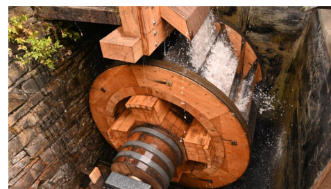
Wasserrad des Hammerwerks in Aktion
